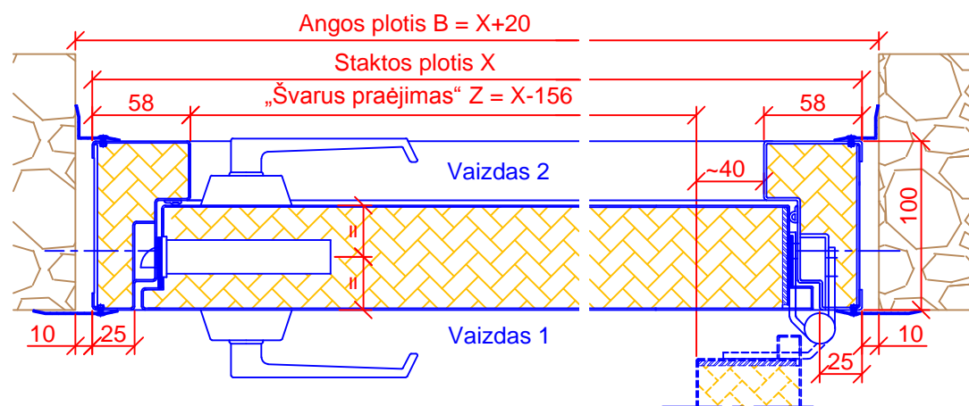
Pjūvis A-A (1:4) Klasikinė stakta
